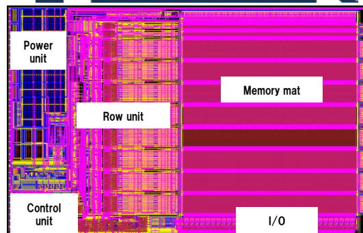
組込フラッシュメモリー回路(フローディア製)
